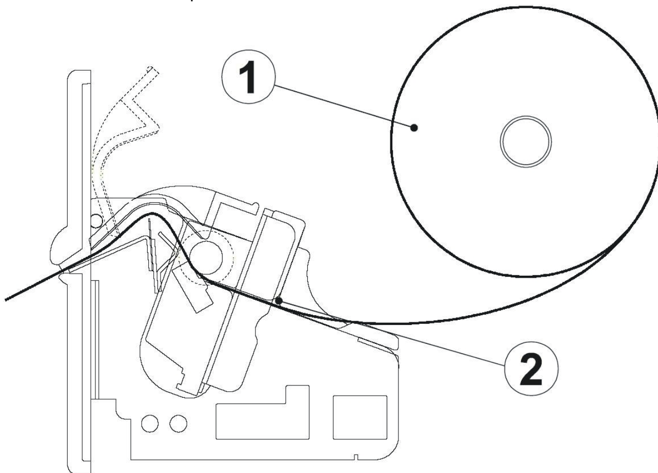
Fig. 3: Cambio rotolo
